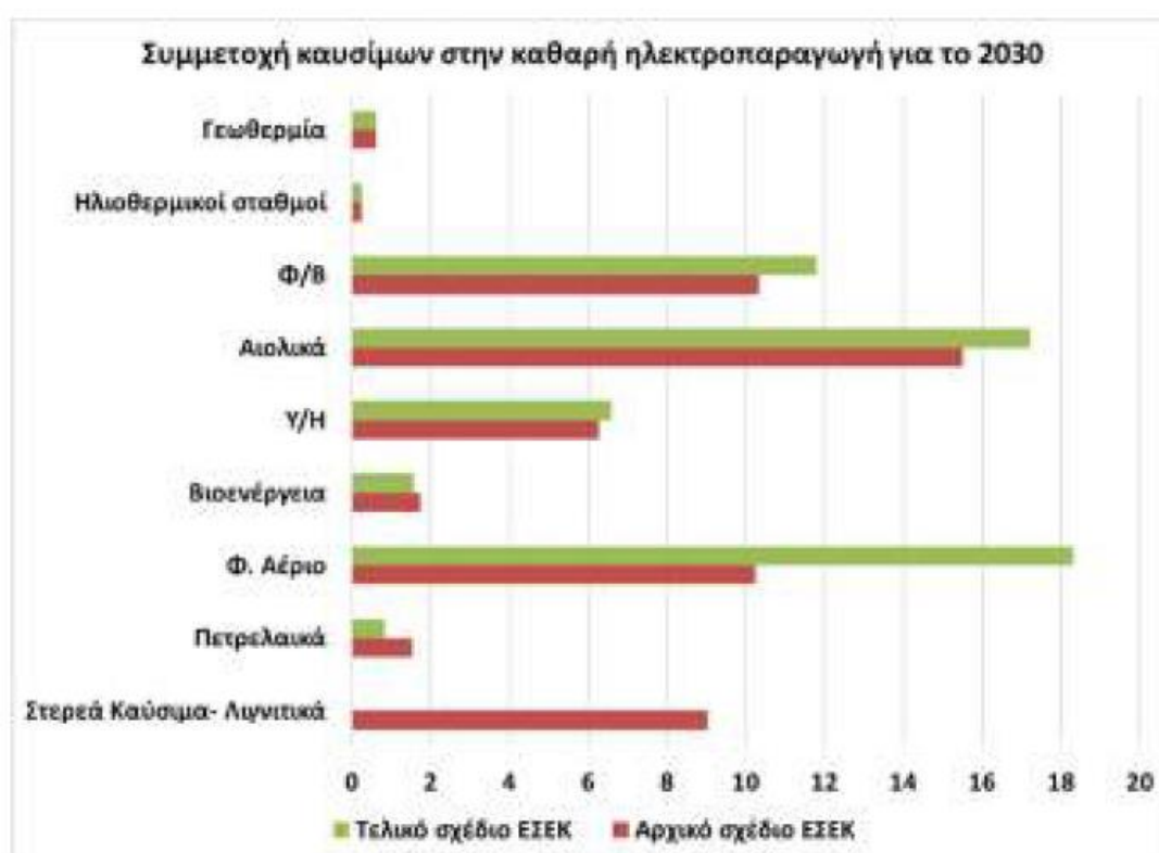
Διάγραμμα 31 - Σύγκριση Συμμετοχής Καυσίμων στη Καθαρή Ηλεκτροπαραγωγή για το 2030, του Αρχικού και Τελικού ΕΣΕΚ
