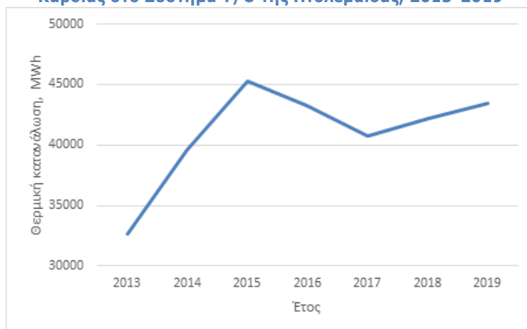
Διάγραμμα 14 - Ετήσια Παροχή Θερμικής Ενέργειας από τις Μονάδες III +IV του ΑΗΣ Καρδιάς στο Σύστημα Τ/Θ της Πτολεμαΐδας, 2013-2019
