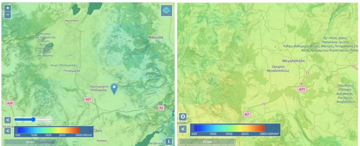
Χάρτης 12 - Ηλιακό Δυναμικό Λιγνιτικών Περιοχών (α) Πτολεμαΐδας-Αμυνταίου (β) Μεγαλόπολης – Μέση Ετήσια Προσπίπτουσα Ηλιακή Ακτινοβολία στο Οριζόντιο Επίπεδο
