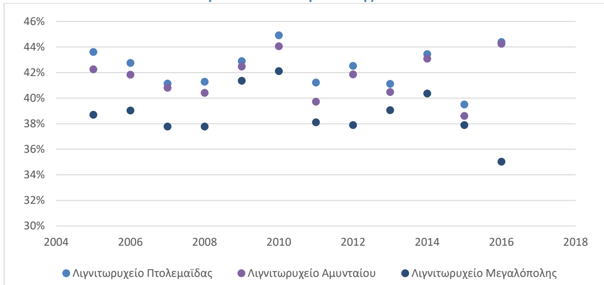
Διάγραμμα 14 - Μέση Τιμή του Λόγου της Διάχυτης Ακτινοβολίας Προς την Ολική (Παγκόσμια) Ηλιακή Ακτινοβολία στο Οριζόντιο Επίπεδο στα Λιγνιτωρυχεία Πτολεμαΐδας, Αμυνταίου και Μεγαλόπολης
