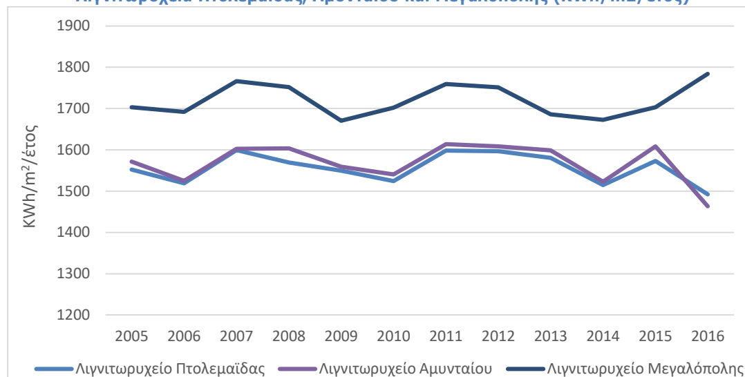
Διάγραμμα 12 - Μέση Ολική Προσπίπτουσα Ακτινοβολία στο Οριζόντιο Επίπεδο στα Λιγνιτωρυχεία Πτολεμαΐδας, Αμυνταίου και Μεγαλόπολης (KWh/m 2 /έτος) 56
