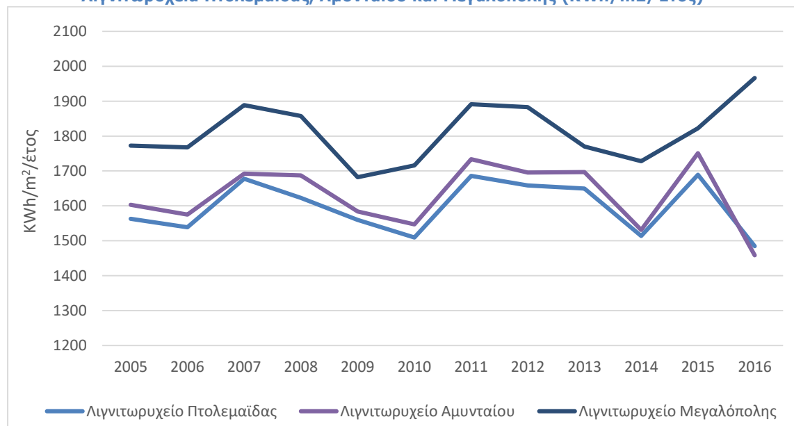
Διάγραμμα 13 - Μέση Προσπίπτουσα Ακτινοβολία Δέσμης στο Οριζόντιο Επίπεδο στα Λιγνιτωρυχεία Πτολεμαΐδας, Αμυνταίου και Μεγαλόπολης (KWh/m 2 /Έτος)
